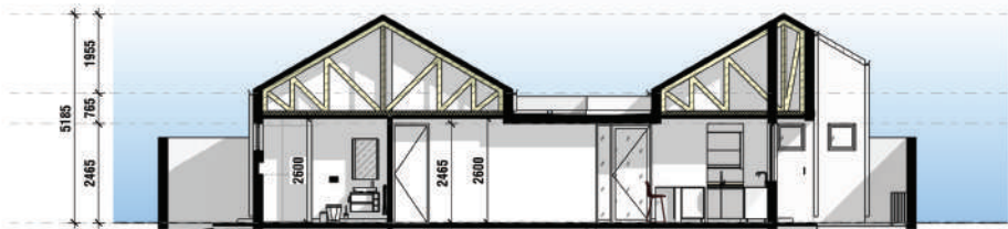
Section 1 SCALE: 1 : 100
