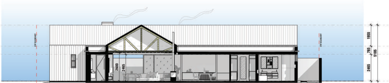
Section 2 SCALE: 1 : 100
