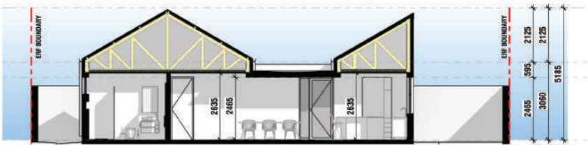
Section 1 SCALE: 1 : 100
