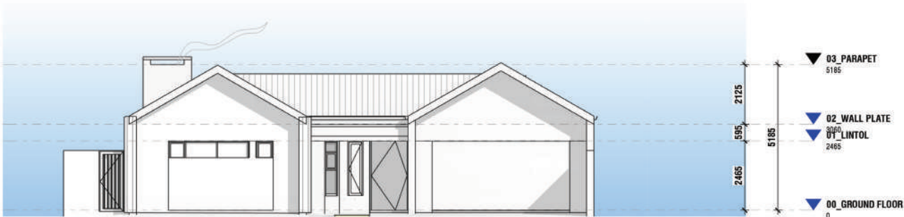
WEST ELEVATION SCALE: 1 : 100
