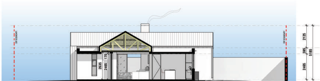
Section 2 SCALE: 1 : 100
