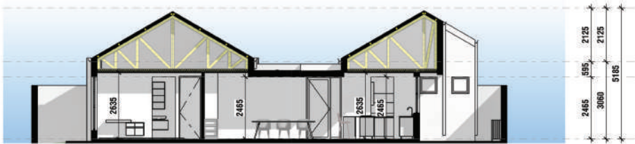
Section 1 SCALE: 1 : 100
