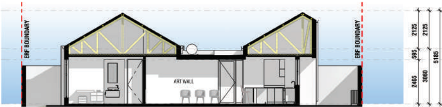
Section 1 SCALE: 1 : 100
