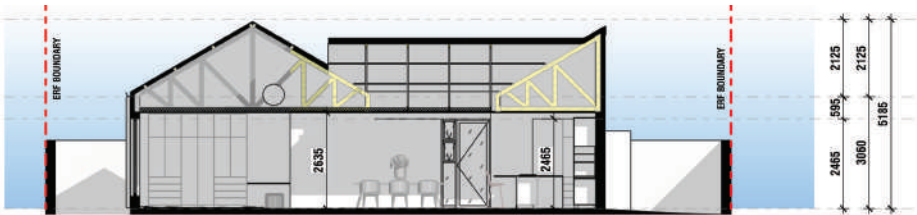
Section 1 SCALE: 1 : 100
