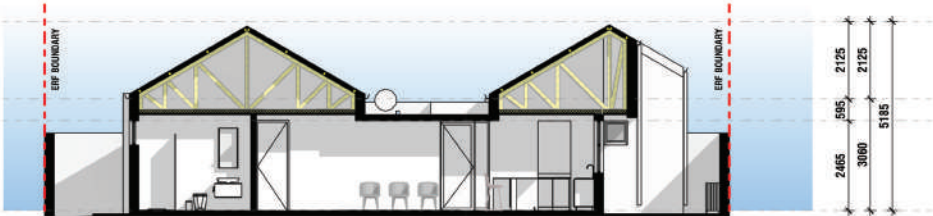
Section 1 SCALE: 1 : 100
