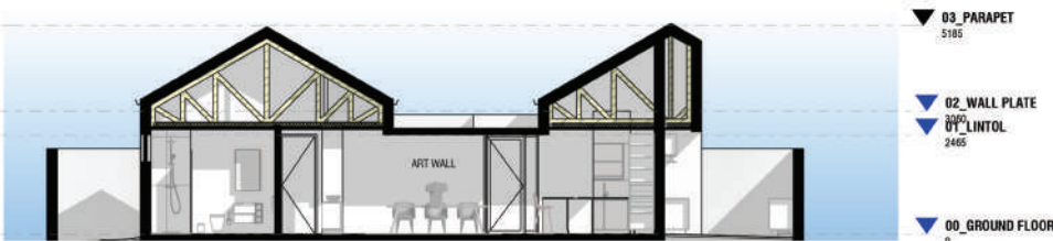
Section 1 SCALE: 1 : 100
