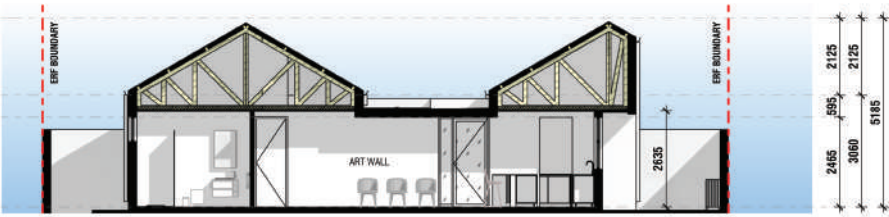
Section 1 SCALE: 1 : 100
