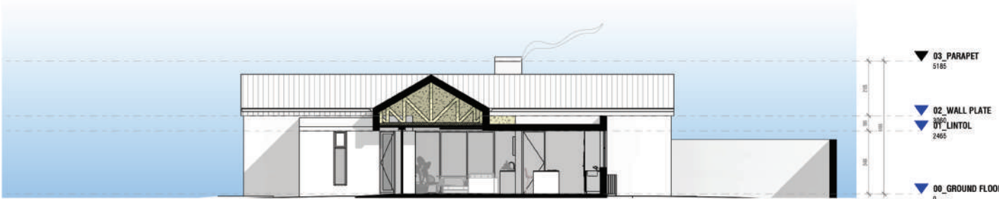
Section 2 SCALE: 1 : 100
