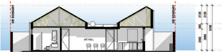
Section 1 SCALE: 1 : 100
